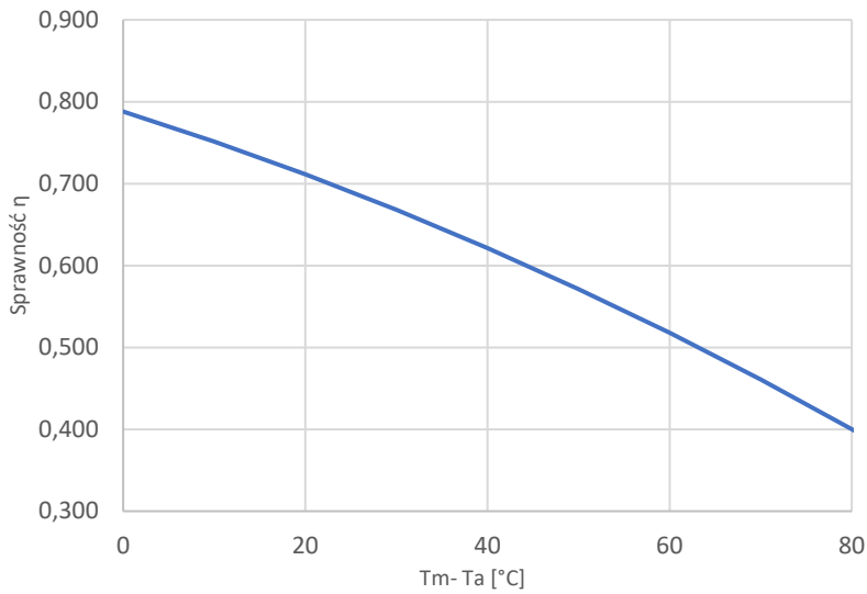
Krzywa sprawności kolektora EM1V/2,0 Al-Cu odniesiona do powierzchni apertury (dla G=1000\text{W/m}^2 )
